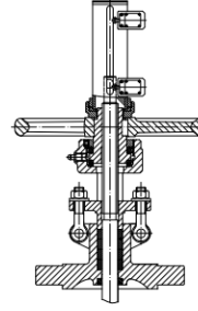
Végálláskapcsoló
