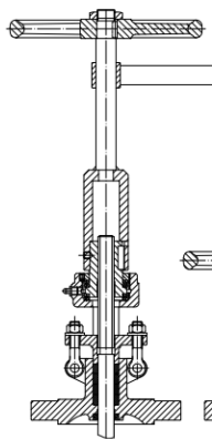
Szárhosszabítással
