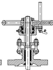
Lakatosható kivitel
